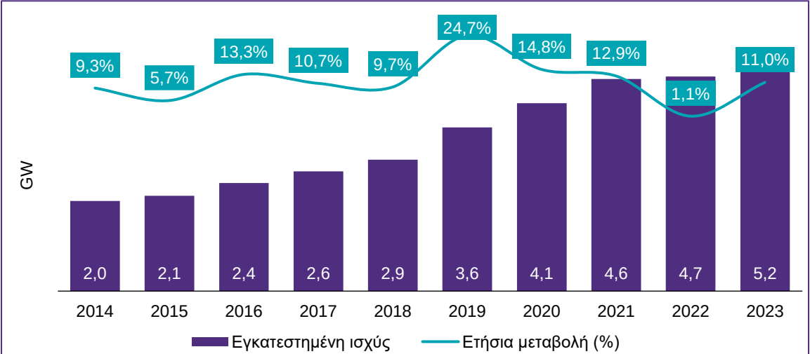
Αιολική ενέργεια | Εγκατεστημένη ισχύς (GW)
