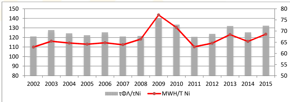
Εικ.4 Εξέλιξη βασικών δεικτών κατανάλωσης (τΦΛ/τNi & MWh/τNi)
