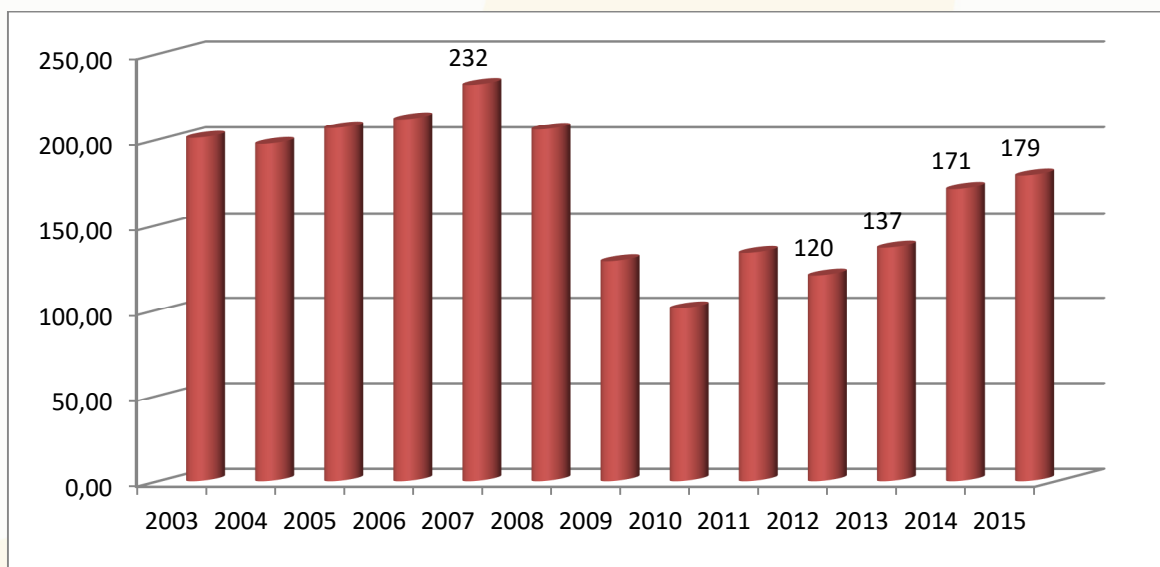
Εικ.5 Εξέλιξη του δείκτη κατανάλωσης των στερεών καυσίμων (kg/τΦΛ)
