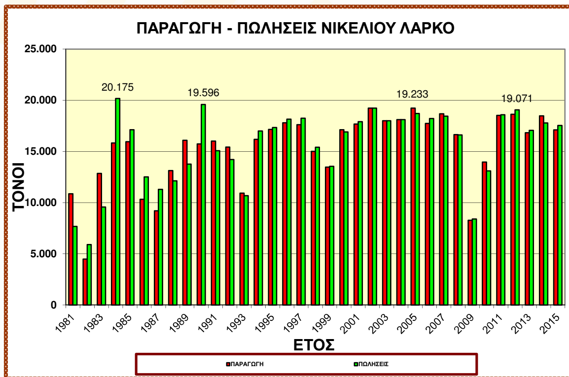
Εικ.3 Εξέλιξη παραγωγής – πωλήσεων Νικελίου σε τόνους Ni
